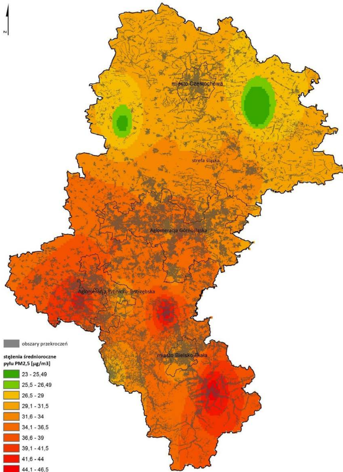
Rysunek 5 Obszary przekroczeń stężeń średniorocznych pyłu zawieszzonego PM 2,5 [źródło: Dwunasta roczna ocena jakości powietrza w województwie śląskim obejmująca 2013 rok, WIOŚ Katowice].
