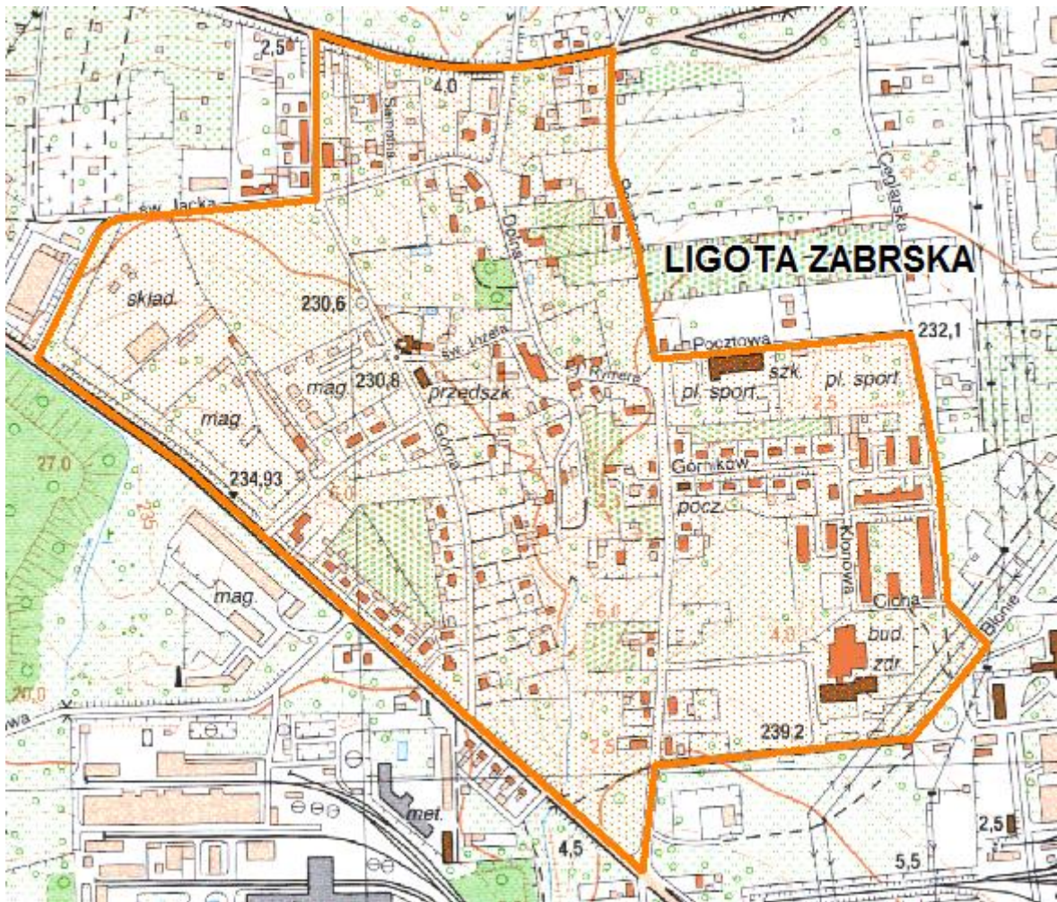
Rysunek 5: Obszar rewitalizacji - Ligota Zabrska
