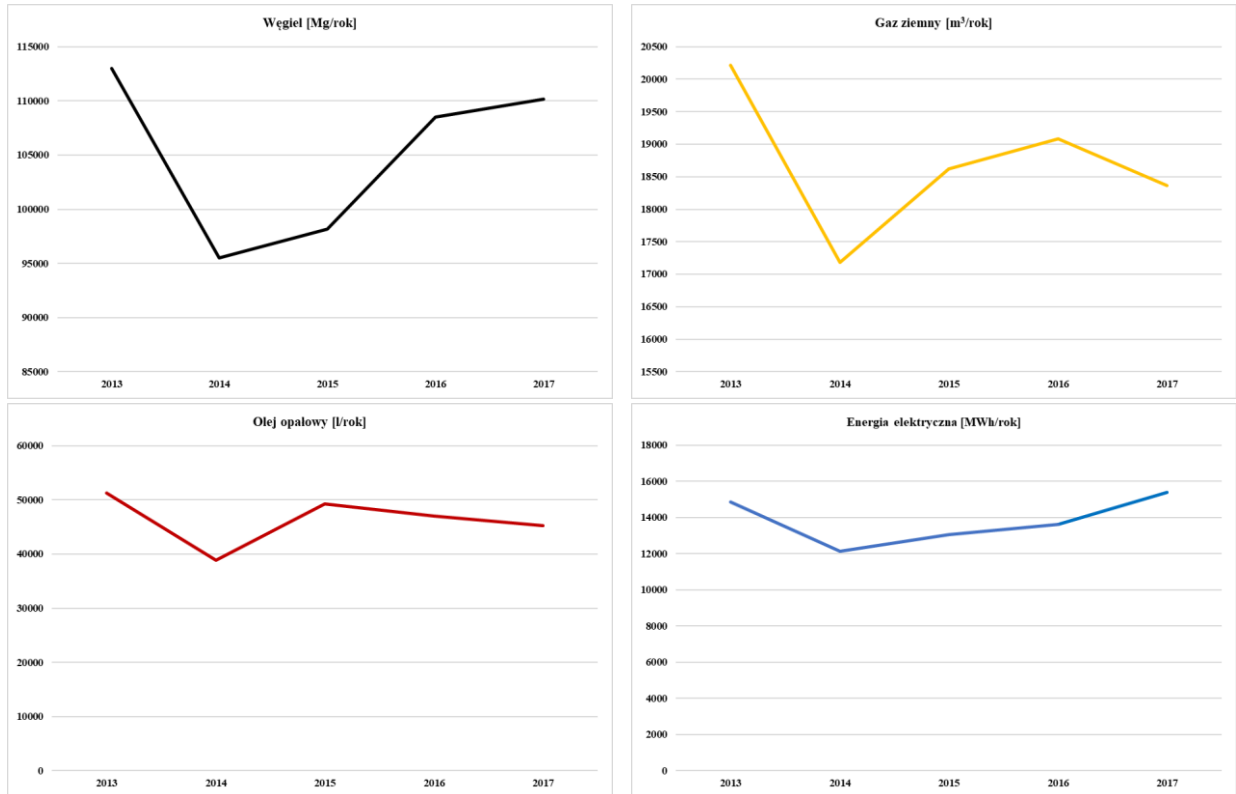
Rys. 7.1. Zużycie paliw w źródłach ciepła PEC - Gliwice Sp. z o.o. w latach 2013÷2017 źródło: Opracowanie własne na podstawie danych PEC - Gliwice Sp. z o.o.
