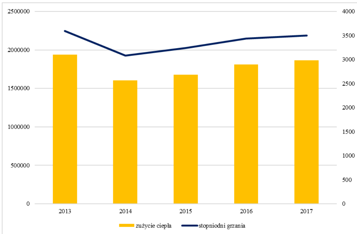
Rys. 7.6. Ciepło dostarczone odbiorcom PEC - Gliwice Sp. z o.o. [GJ/rok] źródło: Opracowanie własne na podstawie danych PEC - Gliwice Sp. z o.o.
