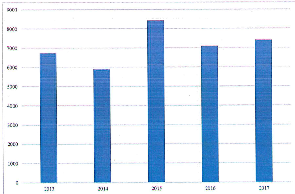
Rys. 8.6. Emisja CO 2 w sektorze oświetlenia [Mg/rok]
