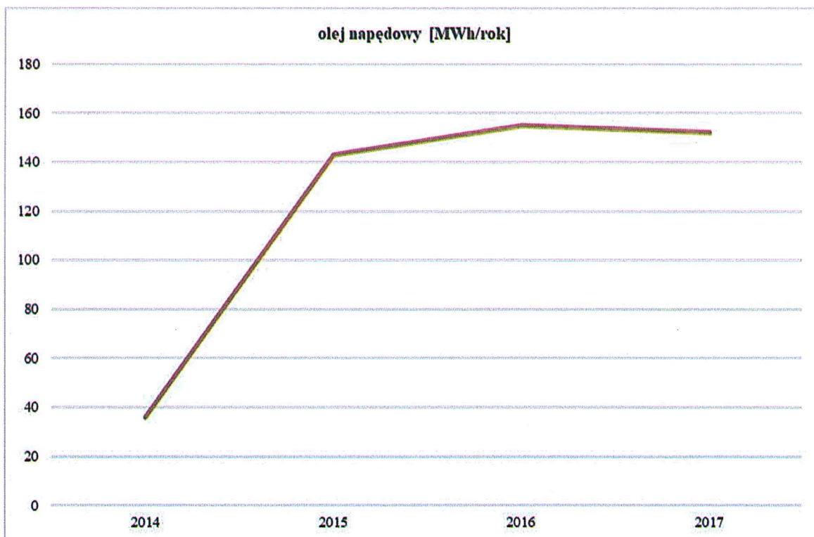
Rys. 7.25. Zużycie paliw przez pojazdy INTER na terenie Gliwic w latach 2014÷2017
