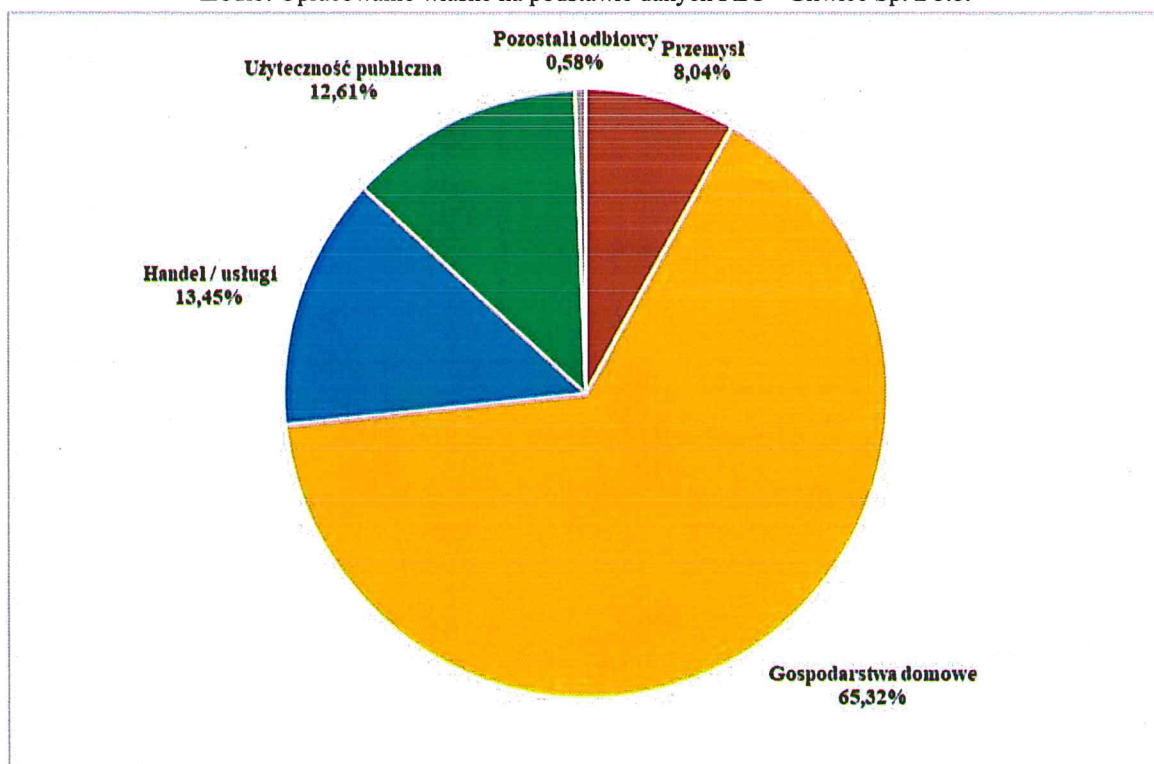
Rys. 7.7. Struktura zużycia ciepła w poszczególnych grupach odbiorców w 2017 roku
