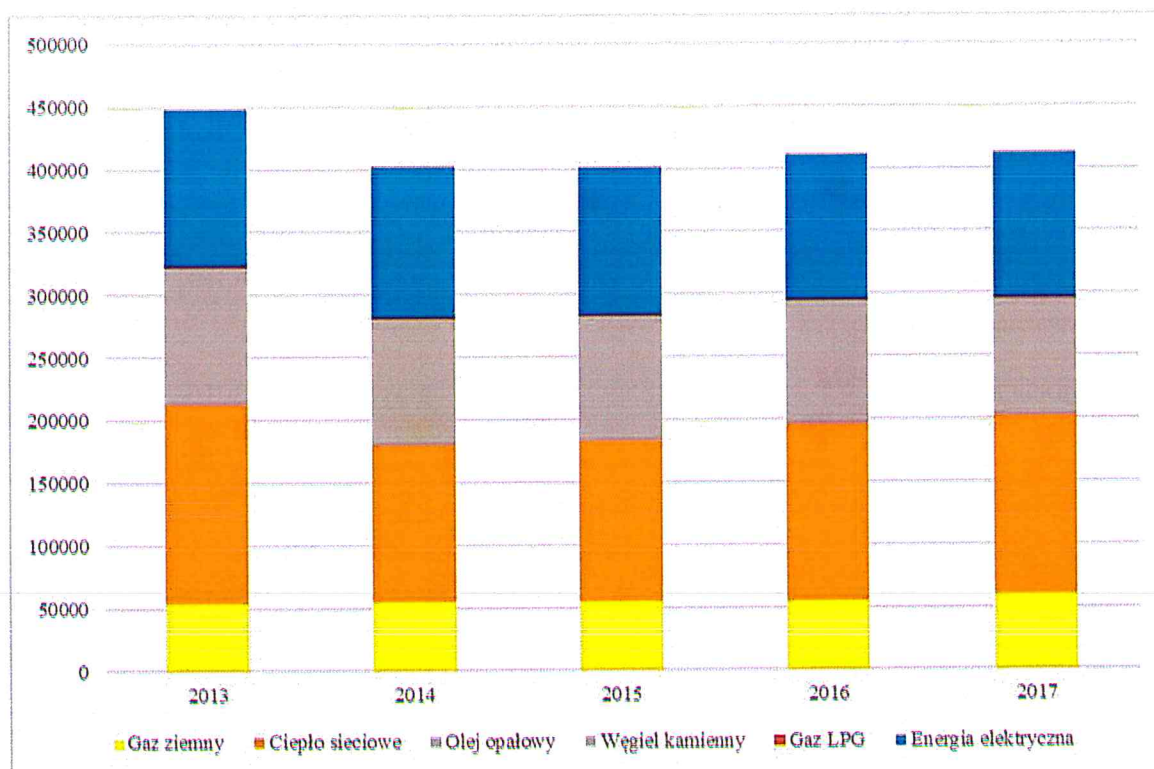
Rys. 8.1. Emisja CO 2 w sektorze budynków mieszkalnych [Mg/rok] źródło: opracowanie własne
