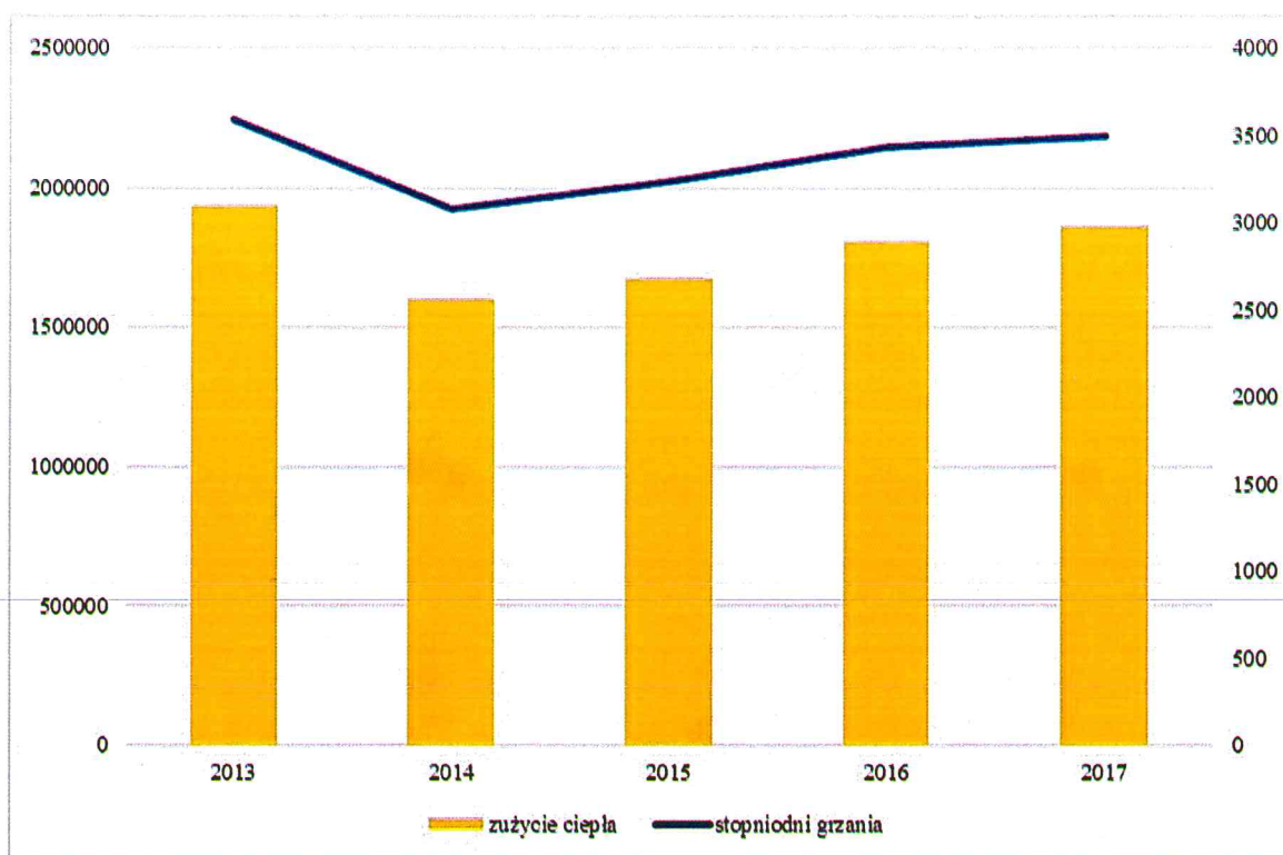
Rys. 7.6. Ciepło dostarczone odbiorcom PEC - Gliwice Sp. z o.o. [GJ/rok]
