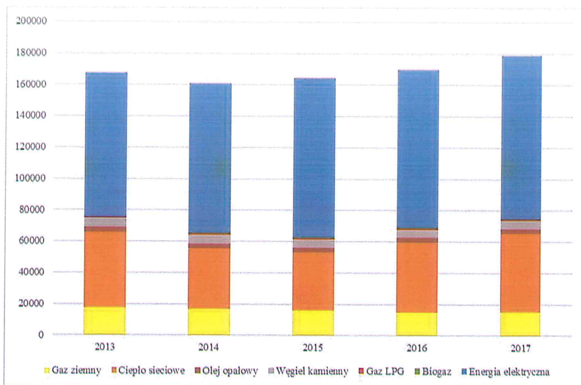
Rys. 8.3. Emisja CO 2 w sektorze handlu i usług [Mg/rok] źródło: opracowanie własne
