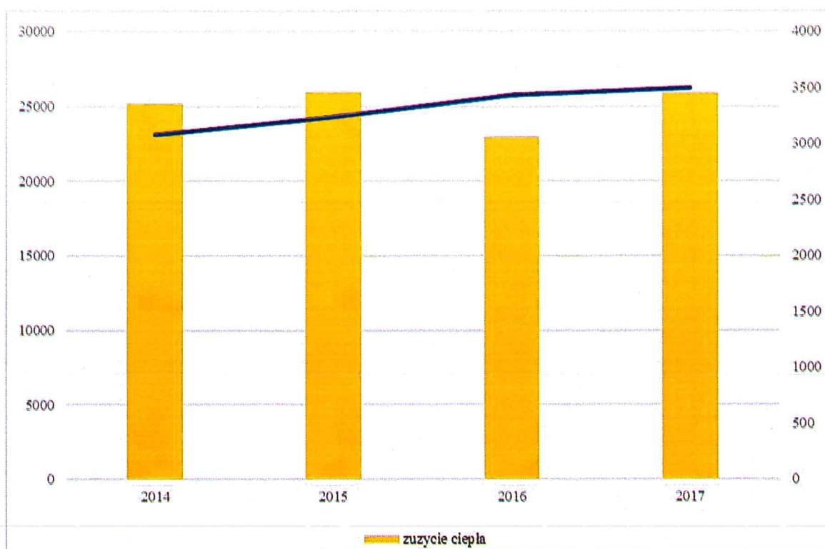
Rys. 7.13. Ciepło dostarczone odbiorcom ZEM Łabędy Sp. z o.o. [GJ/rok]
