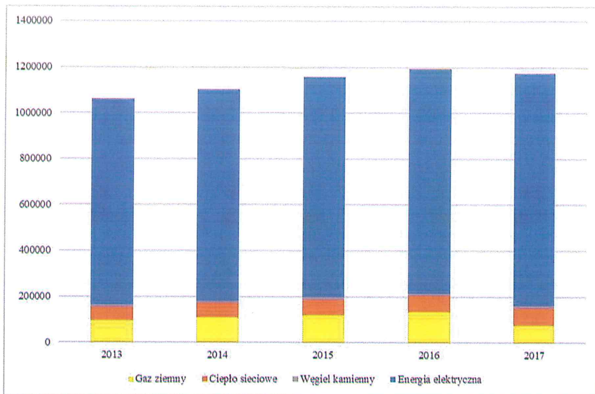
Rys. 8.4. Emisja CO 2 w sektorze przemysłu [Mg/rok]
