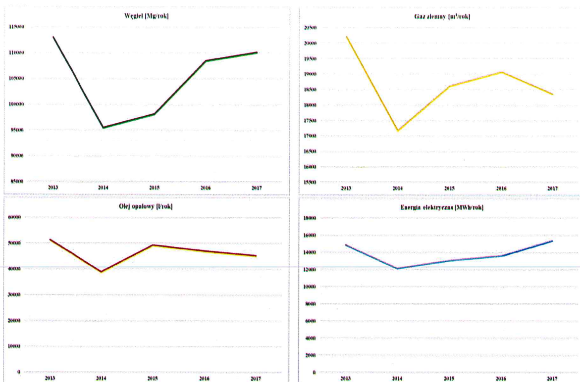
Rys. 7.1. Zużycie paliw w źródłach ciepła PEC - Gliwice Sp. z o.o. w latach 2013÷2017 źródło: Opracowanie własne na podstawie danych PEC - Gliwice Sp. z o.o.
