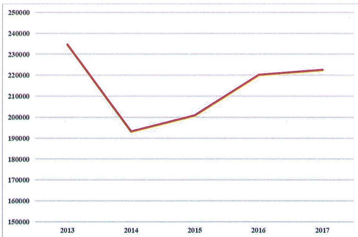
Rys. 7.3. Emisja CO 2 ze źródeł ciepła PEC - Gliwice Sp. z o.o. [Mg/rok] źródło: Opracowanie własne na podstawie danych PEC - Gliwice Sp. z o.o.
