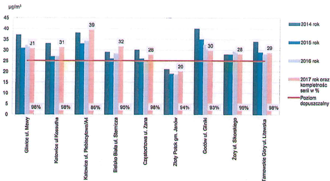
Rys. 5.23. Średnie roczne stężenia pyłu PM 2,5 w latach 2014-2017
