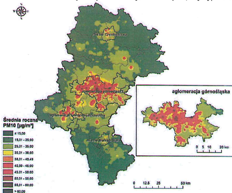
Rys. 5.26. Obszary przekroczeń średnich stężeń rocznych pyłu zawieszonego PM10 źródło: Szesnasta roczna ocena jakości powietrza w województwie śląskim, obejmująca 2017 rok
