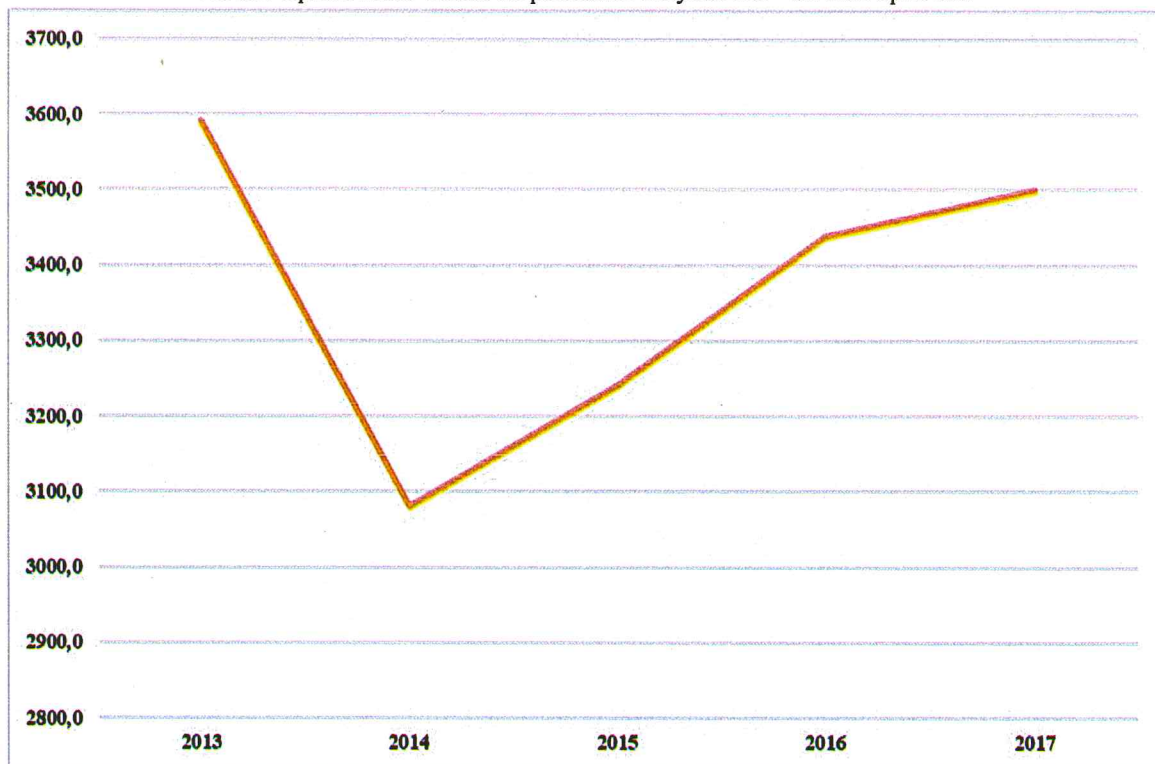
Rys. 7.2. Liczba stopniodni grzania w latach 2013÷2017 w województwie śląskim źródło: Opracowanie własne na podstawie danych GUS
